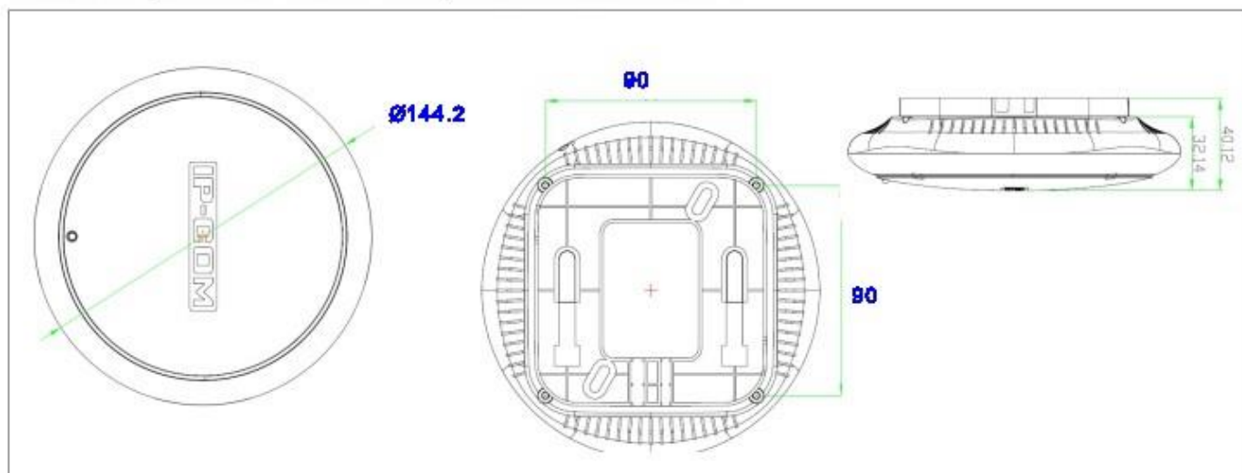
圖2: 產品結構線框圖
